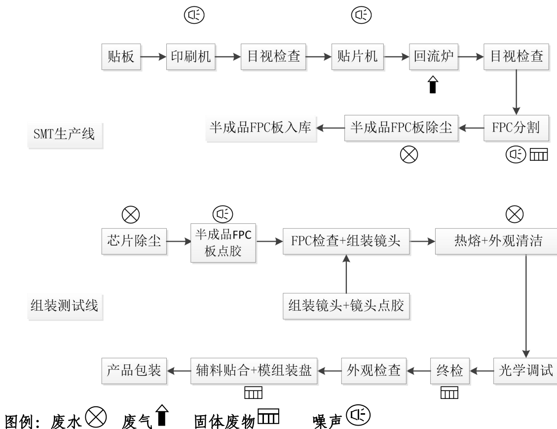
图 3.1.5-1 项目生产工艺流程图
