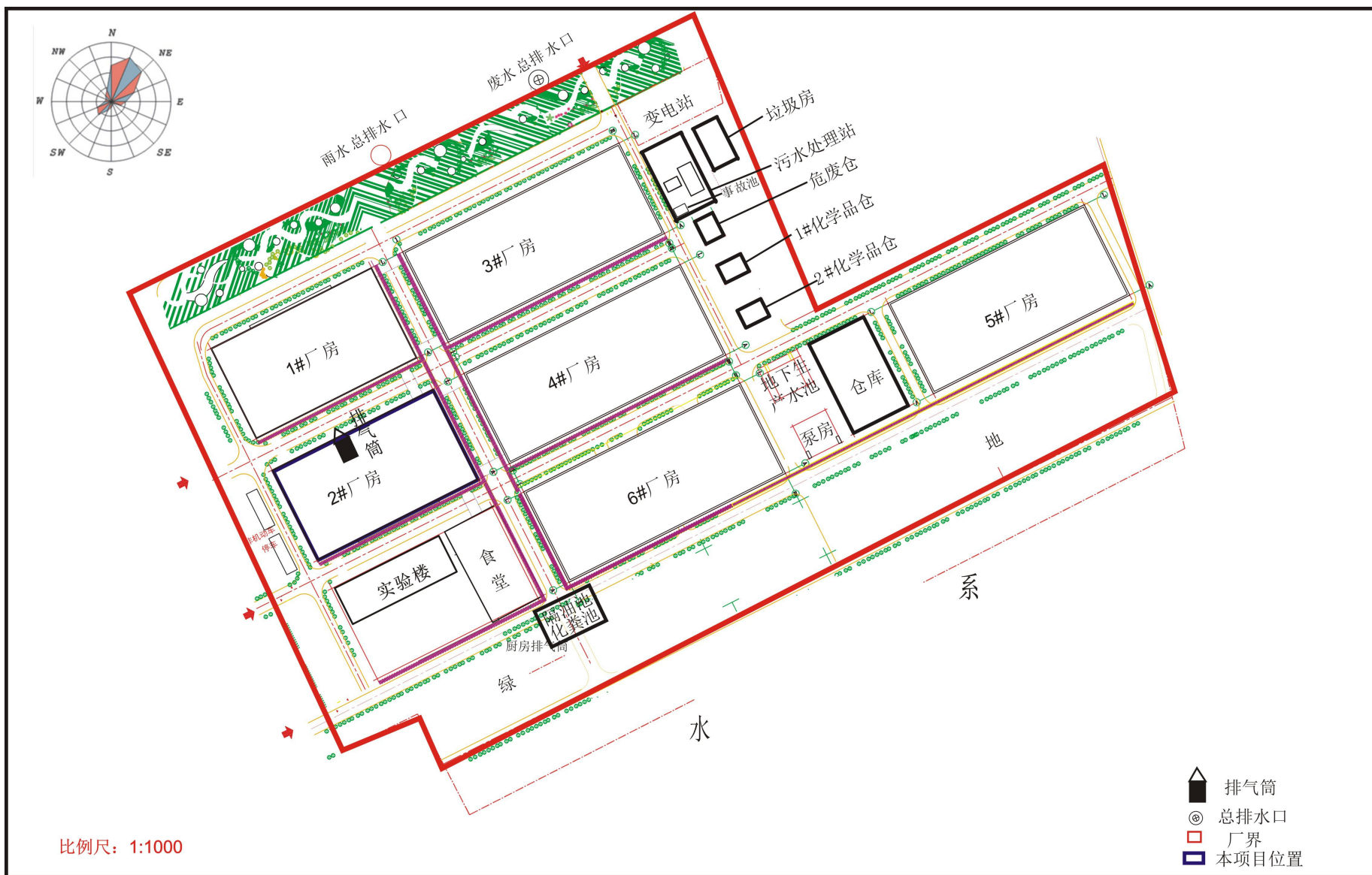
附件 3: 项目所在园区平面布置图
