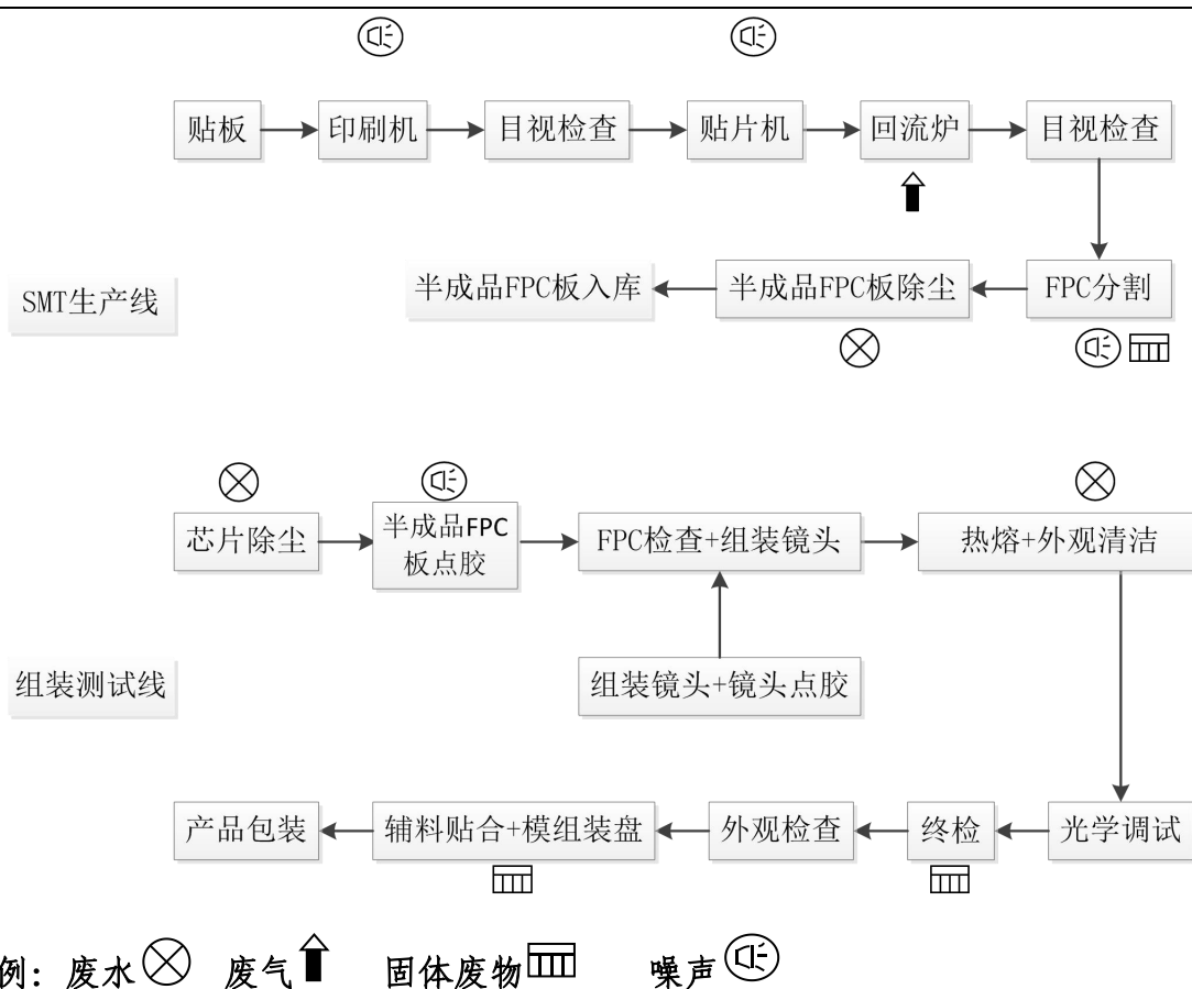
图 2.4.1-1 项目生产工艺流程图
